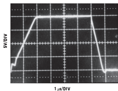
LF356
