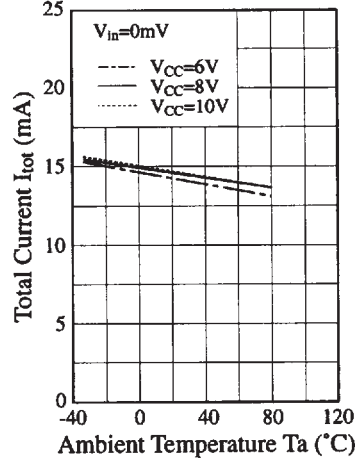
I_{tot} - T_a
