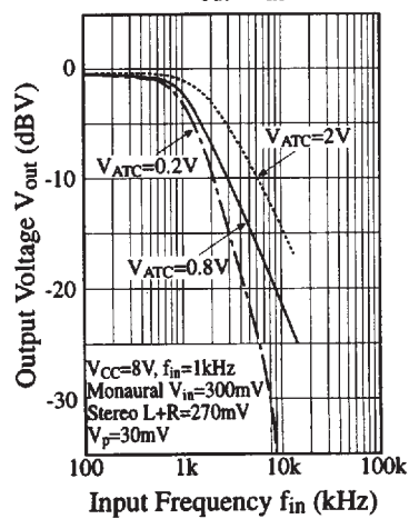
V_{out} - f_{in}
