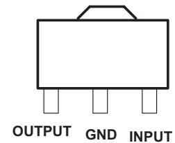
SOT-89 78L06CPK
