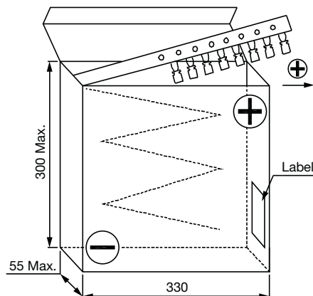
Fig. 5 - Ammopack box
