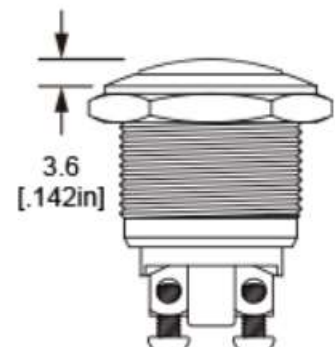
Domed Actuator
