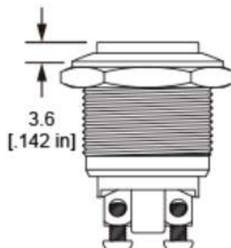
High Actuator
