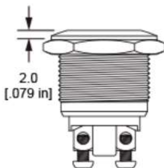
Flat Actuator
